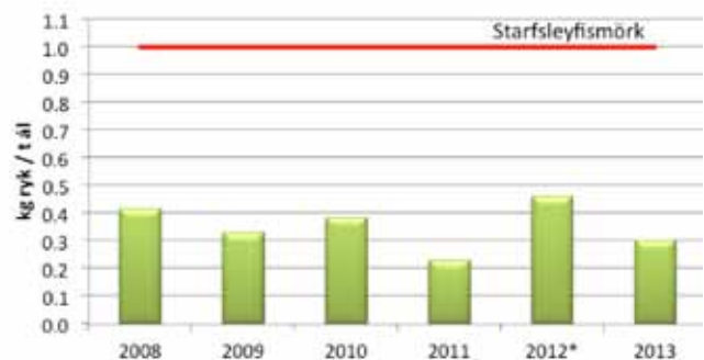
Mynd 3 Losun ryks árin 2008 til 2013.
