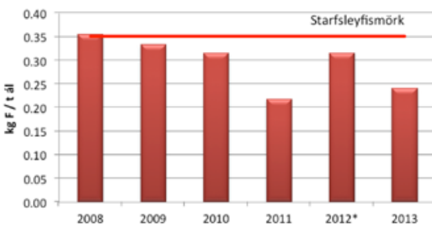
Mynd 2 Losun heildarflúoríðs árin 2008 til 2013
