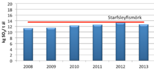
Mynd 4 Losun brennisteinsdíoxíðs frá forskautum árin 2008 til 2013.
