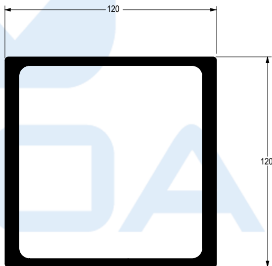
CA-356 8,096 kg/m Fueiro
