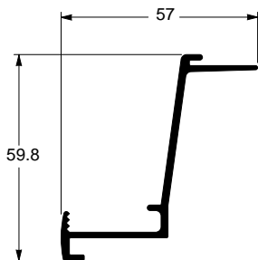
TP-0847 0,621 kg/m Moldura para porta
