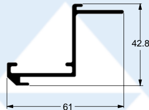
CA-176 0,684 kg/m Moldura para porta
