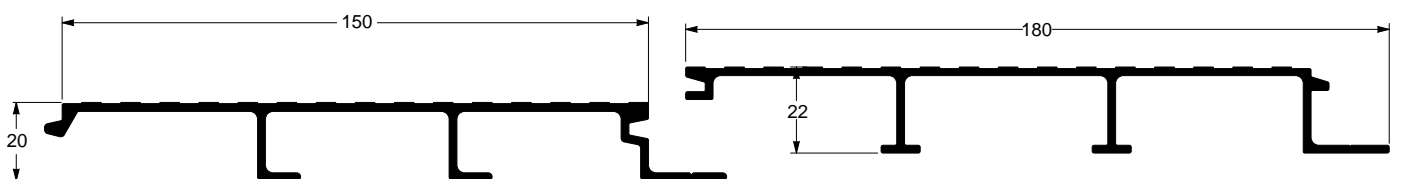
CA-0308 1,507 kg/m Piso carroceria seca
