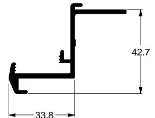
TP-0084 0,749 kg/m Moldura para porta
