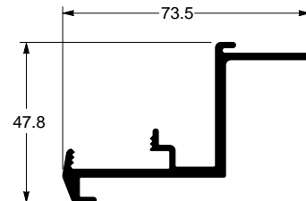
TP-720 0,987 kg/m Moldura para porta
