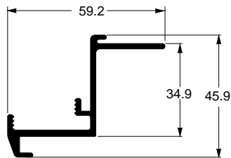
CA-0307 0,736 kg/m Moldura para porta
