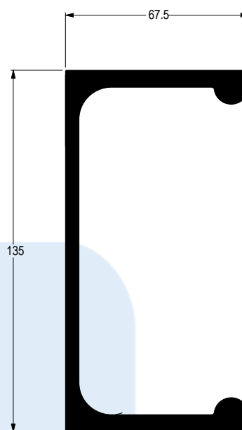
CA-327 4,491 kg/m Travessa da base
