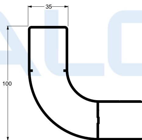
CA-0736 1,927 kg/m Remate do paraciclo
