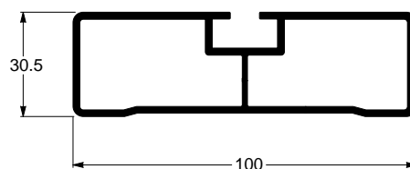
CA-0737 1,617 kg/m Grade do paraciclo
