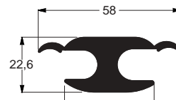
EE-1808 1,353 kg/m
