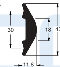
EE-1385 0,745 kg/m
