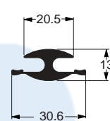
EE-0743 0,393 kg/m Conector elétrico
