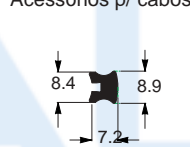
EE-0663 0,133 kg/m Separador elétrico
