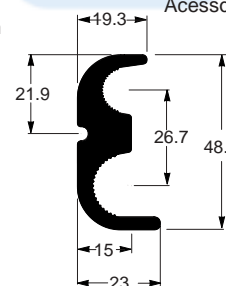
EE-1558 1,211 kg/m Conector elétrico
