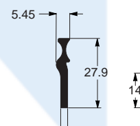
EE-0637 0,225 kg/m Separador conector
