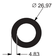
TR-1084 0,910 kg/m Tubo redondo
