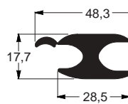
EE-1825 0,868 kg/m
