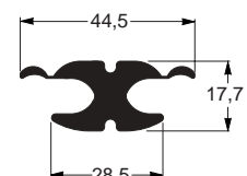
EE-1347 0,865 kg/m
