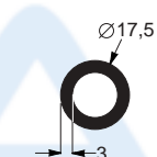
TR-1082 0,371 kg/m Tubo redondo
