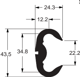
EE-0747 1,103 kg/m Corpo
