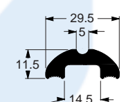
DS-0037 0,490 kg/m Acessório p/ cabos
