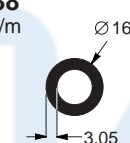
TR-1089 0,336 kg/m Tubo redondo
