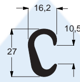
EE-0661 0,470 kg/m
