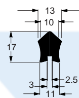
EE-0746 0,381 kg/m Separador elétrico
