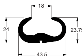
EE-0659 1,060 kg/m Corpo elétrico
