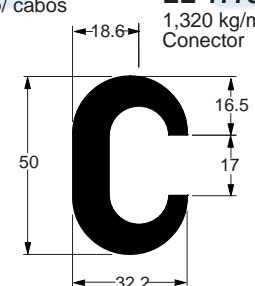
EE-1553 0,556 kg/m
