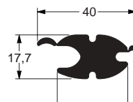
EE-1824 0,975 kg/m
