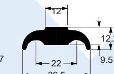
EE-0657 0,645 kg/m Conector eletrônico
