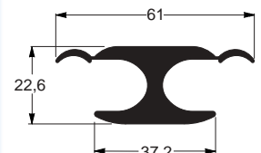
EE-0707 1,138 kg/m
