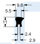
EE-0660 0,179 kg/m Separador
