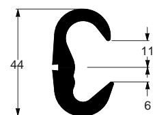
EE-0750 1,197 kg/m Corpo
